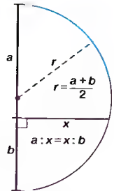
Пропорція Побудова відрізка, який задовольняє пропорції a : x = x : b
